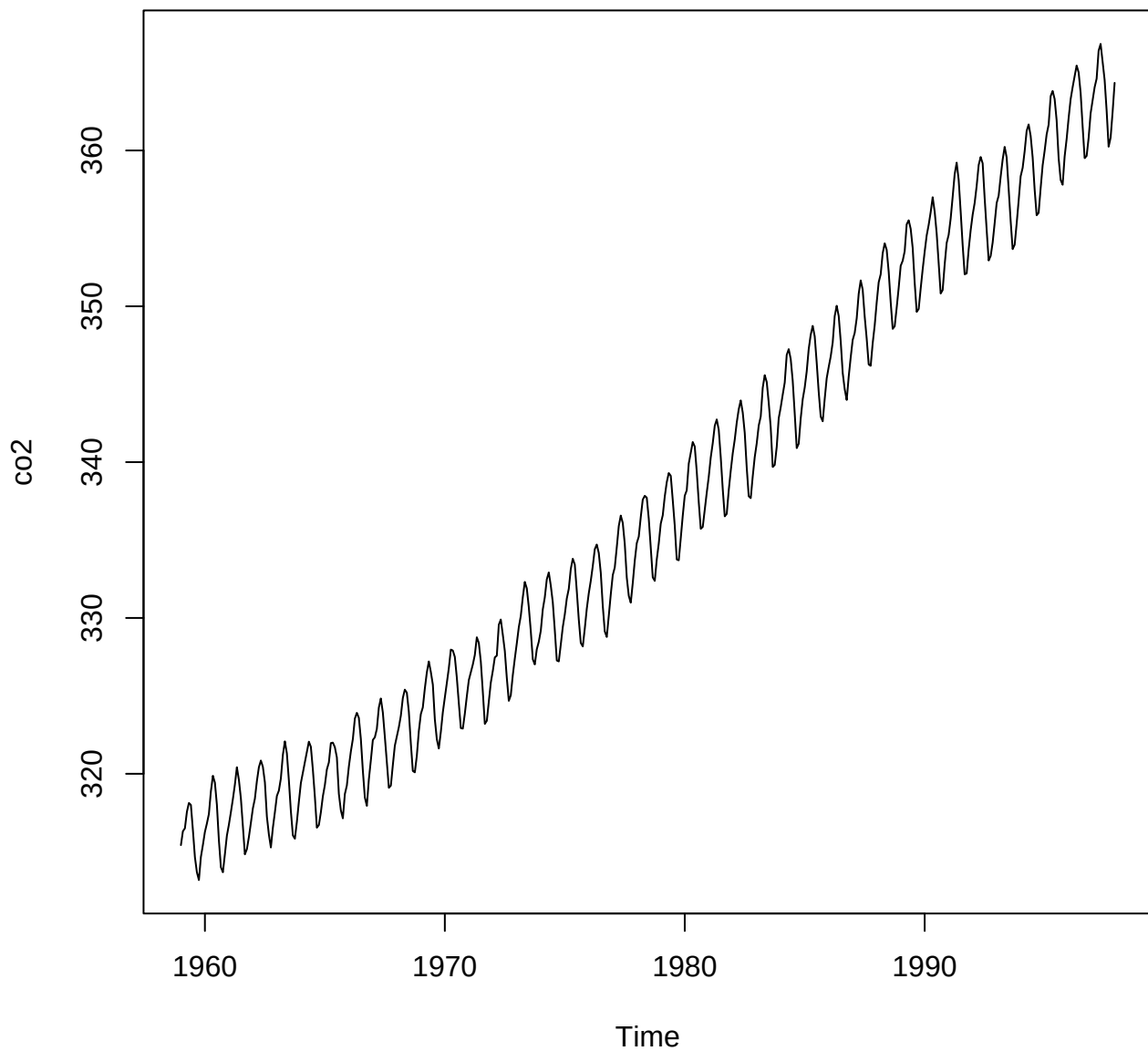
CO2 Mauna Loa (1959–1997)
